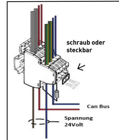
Detailzeichnung Anschluss Doppelstockklemme
